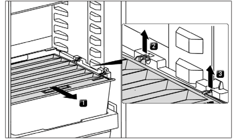
Fig. 8.11 Retirer le couvercle de contrôle de l'humidité
